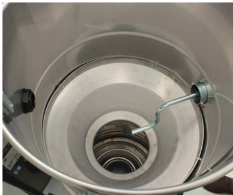
Sacudidor de filtro manual (vista interna)
